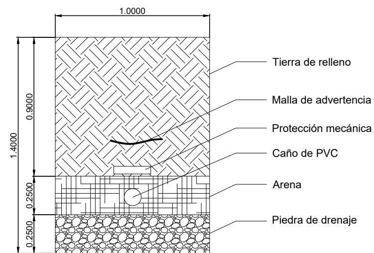
CORTE A-A DETALLE DE EXCAVACIÓN UN CAÑO
