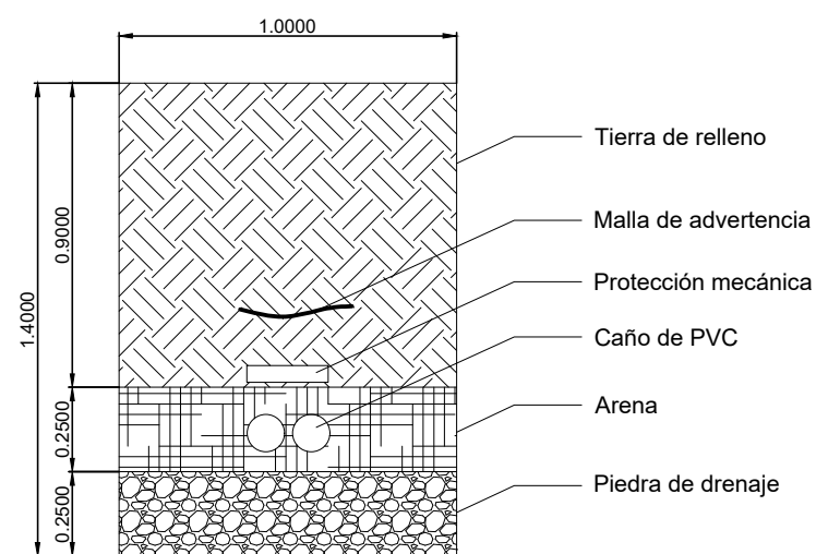
CORTE B-B DETALLE DE EXCAVACIÓN DOS CAÑOS
